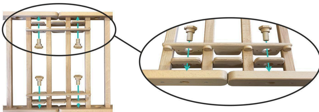
Ukázka montáže spojky E1 pro spojení dvou panelů.
